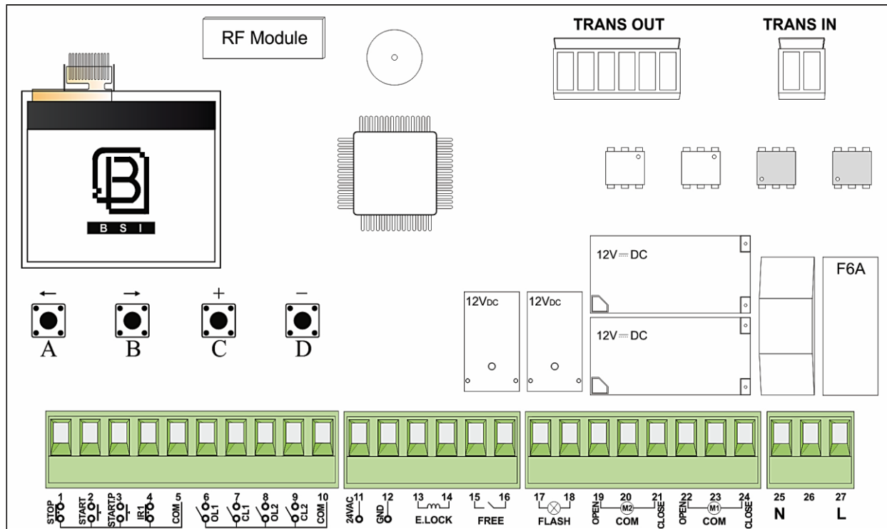
۸-۱. ترمینال‌های ورودی و خروجی مدار کنترل
